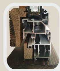
Dettaglio Nodo
